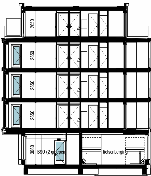
doorsnede B
